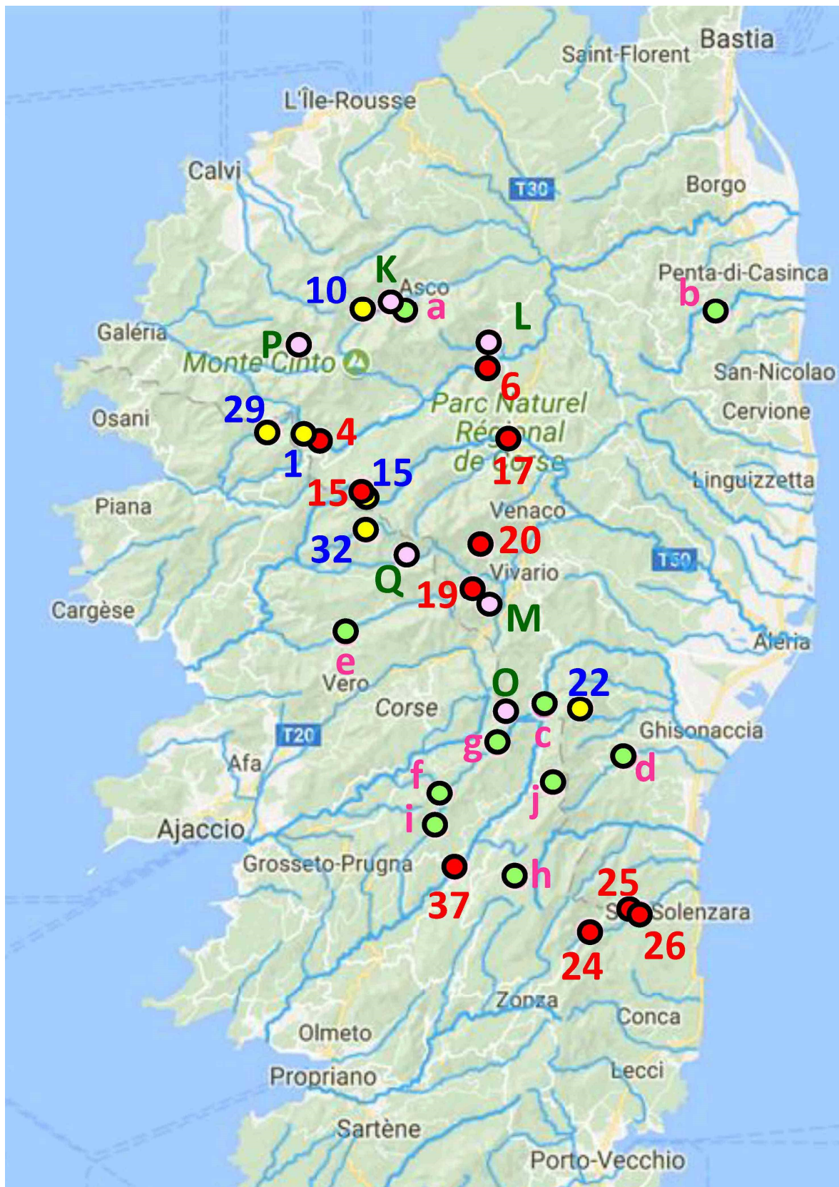
Figure 1: Distribution des stations utilisées dans la méta-analyse: - chiffres rouges sur ronds rouges = allozymes sur méditerranéennes - chiffres bleus sur ronds jaunes = microsatellites sur méditerranéennes - lettres minuscules roses sur rond vert = allozymes sur corses - lettres majuscules vertes sur ronds roses = microsatellites sur corses
